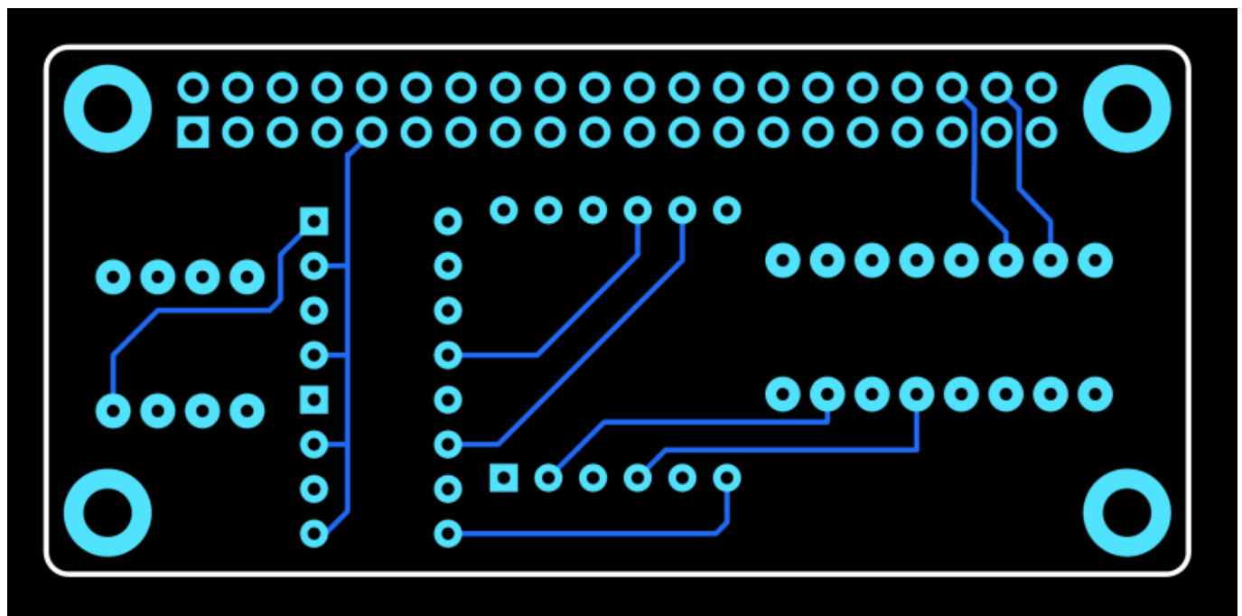
Bottom Layer Copper
