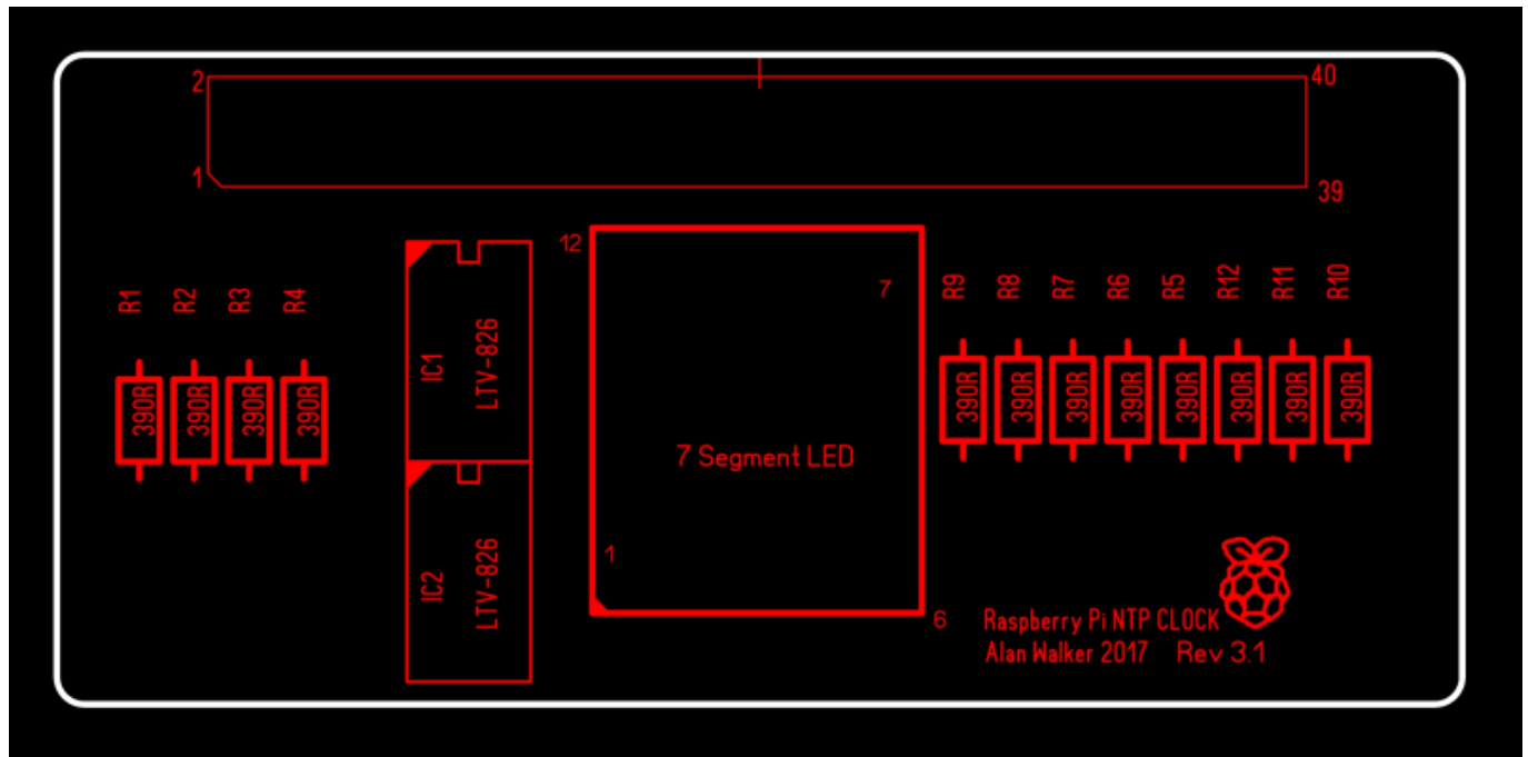
Top Layer Copper
